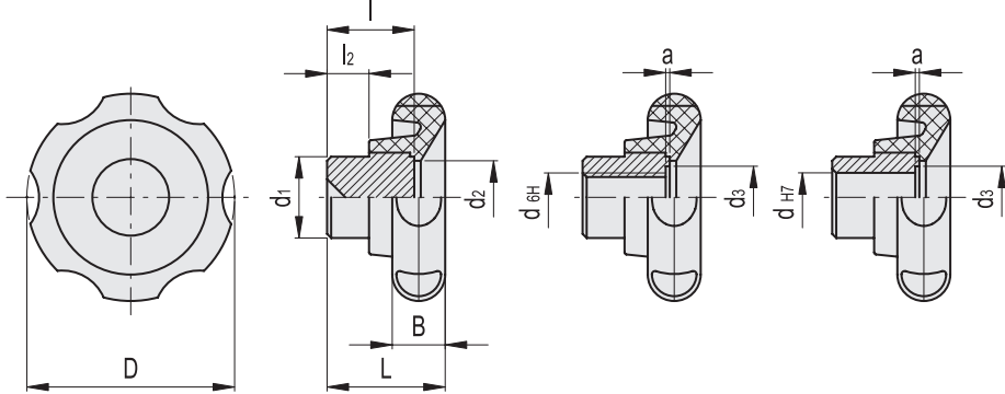
VL.640-FP VL.640-FP-B
