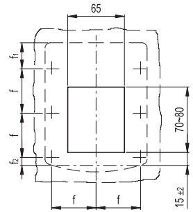
Delik açma şablonu
