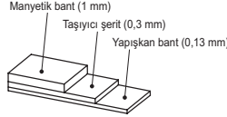
Şekil 3 Doğru montaj
