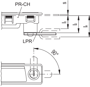
PR-CH kol üzerine montaj
