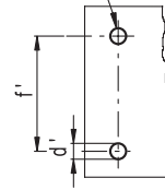
Delme şablonu Çapaksız ve yivsiz delikler
