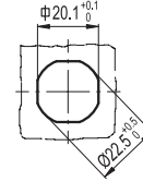
Delik açma şablonu
