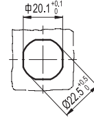
Delik açma şablonu
