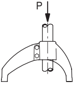
Tutma Kuvveti P = 2000 N
