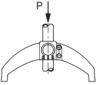
Tutma Kuvveti P = 2000 N
