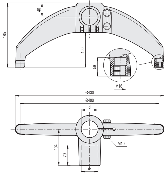
Maksimum statik yük P = 9800 N
